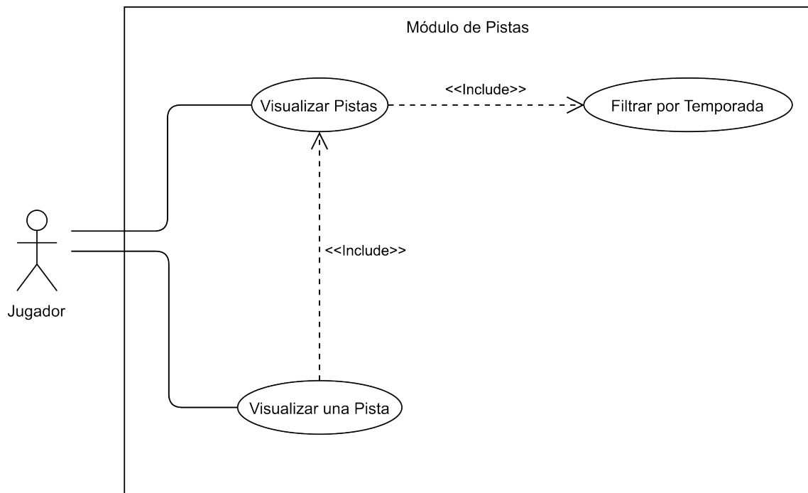
Figura 6.5: Segundo diagrama de casos de uso del módulo de pistas
