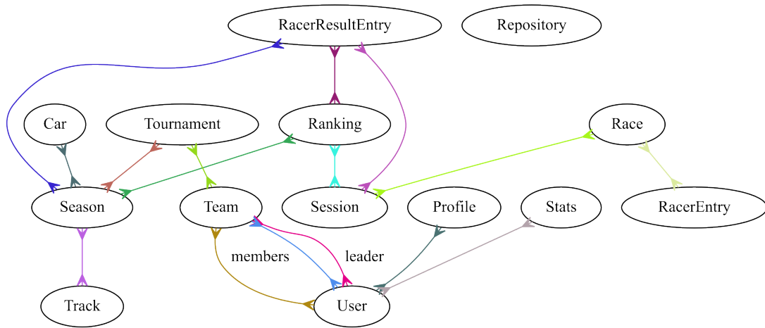
Figura 6.10: Resumen de modelos de datos
