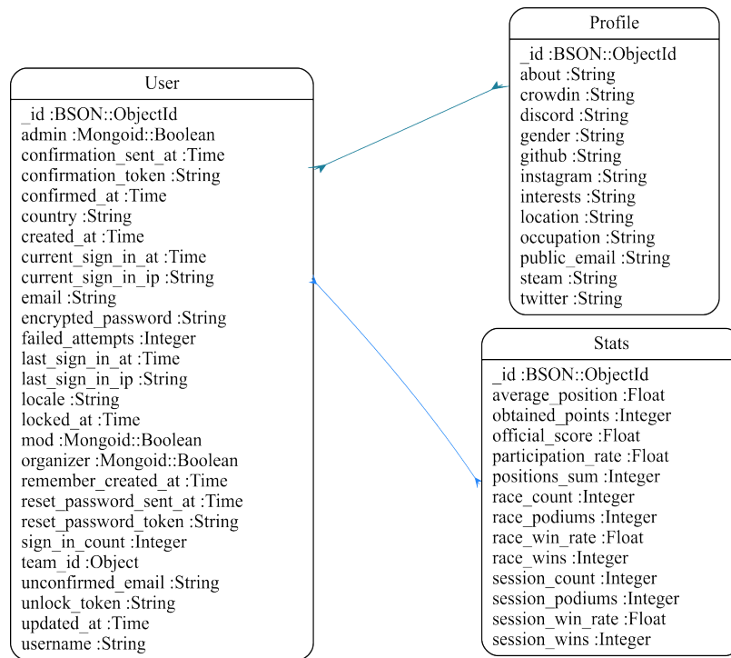
Figura 6.11: Modelo de relaciones entre usuario, perfil y estadísticas
