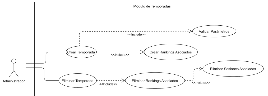
Figura 6.6: Primer diagrama de casos de uso del módulo de temporadas
