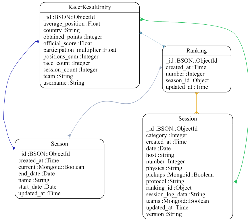
Figura 6.13: Modelo de relaciones entre temporada, ranking y sesiones con sus componentes
