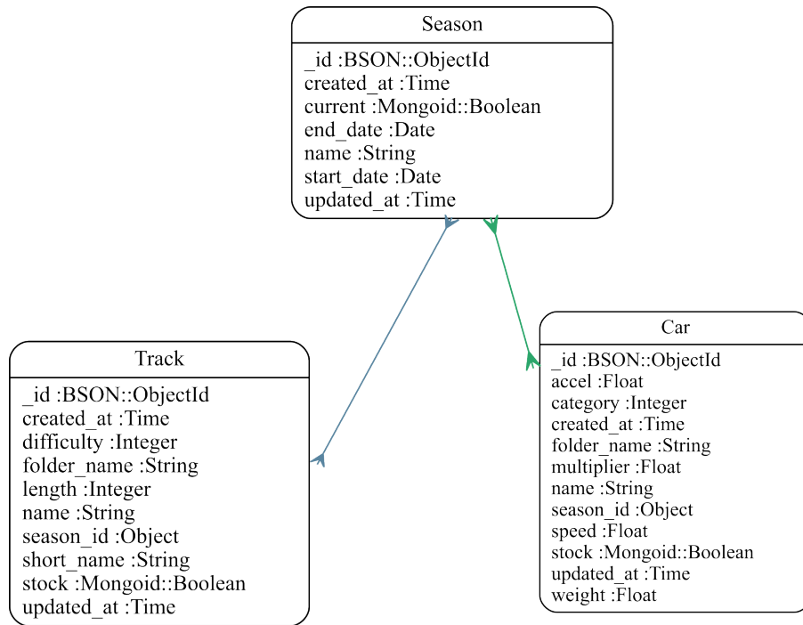
Figura 6.12: Modelo de relación entre temporada, autos y pistas
