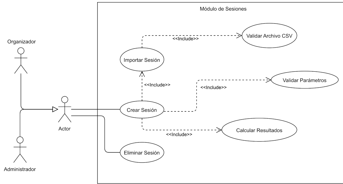
Figura 6.8: Primer diagrama de casos de uso del módulo de sesiones
