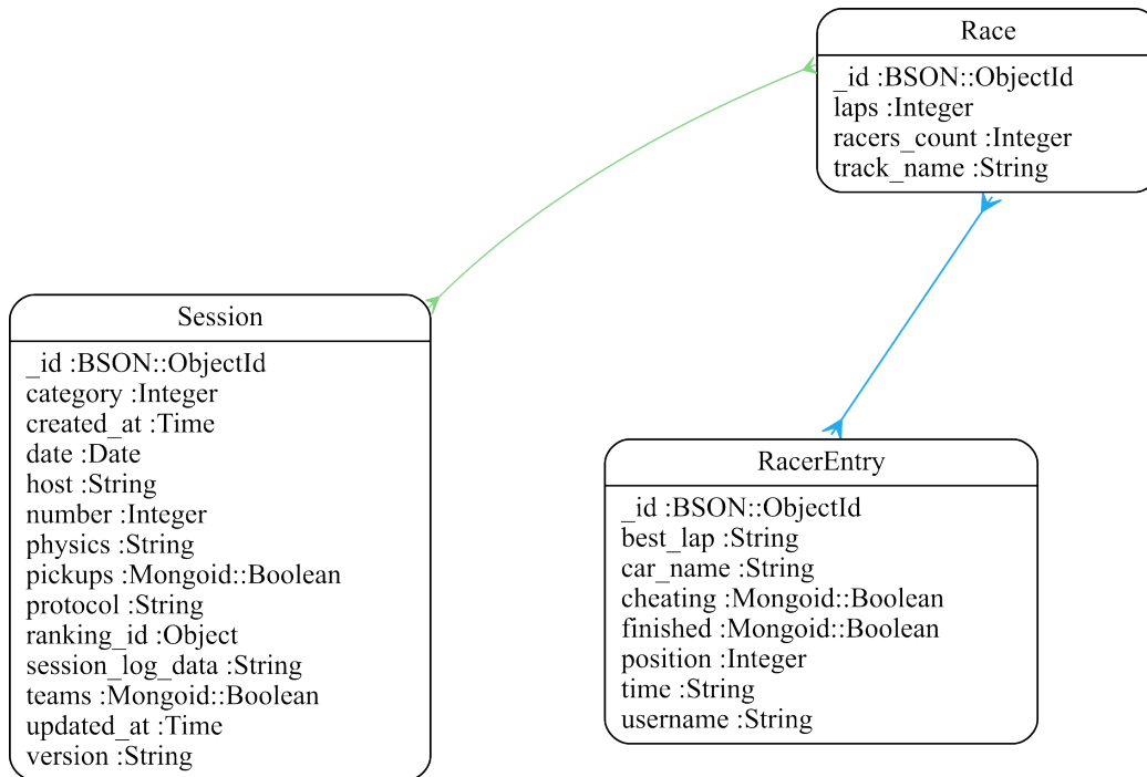
Figura 6.14: Modelo de relación entre sesión, carrera y entrada de corredor
