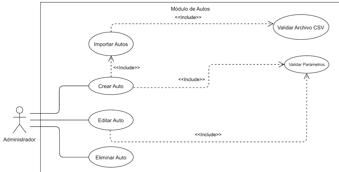
Figura 6.2: Primer diagrama de casos de uso del módulo de autos
