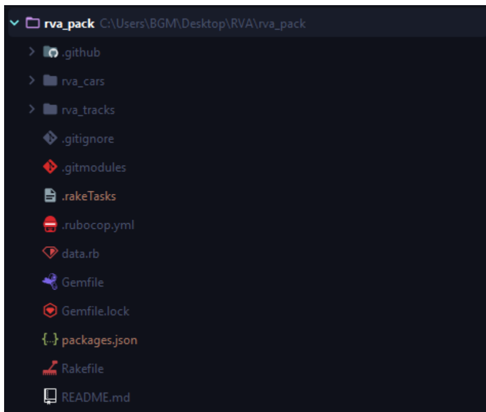
Figura 4.1: Árbol de directorios de rva_pack
