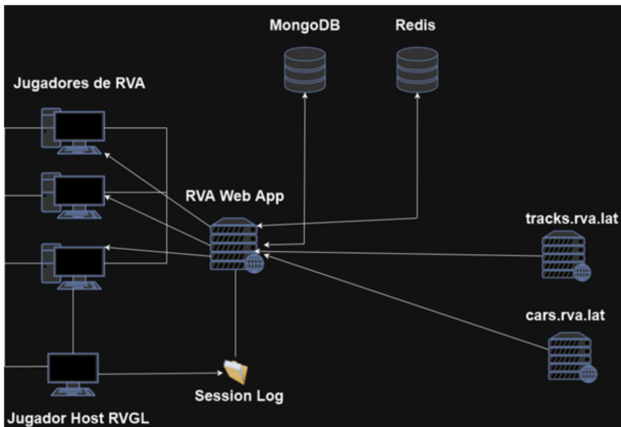
Figura 6.26: Diagrama de arquitectura de RVA
