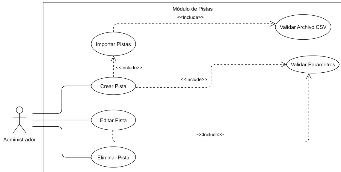
Figura 6.4: Primer diagrama de casos de uso del módulo de pistas
