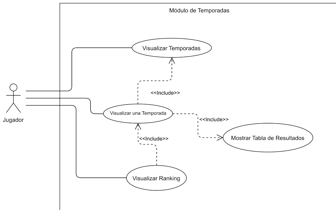
Figura 6.7: Segundo diagrama de casos de uso del módulo de temporadas
