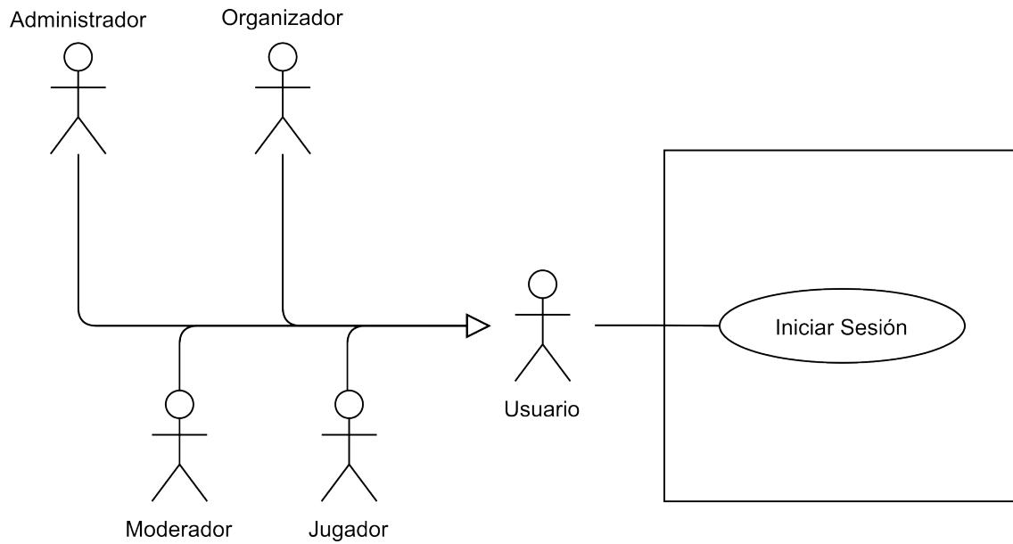
Figura 6.1: Diagrama de casos de uso del módulo de privilegios
