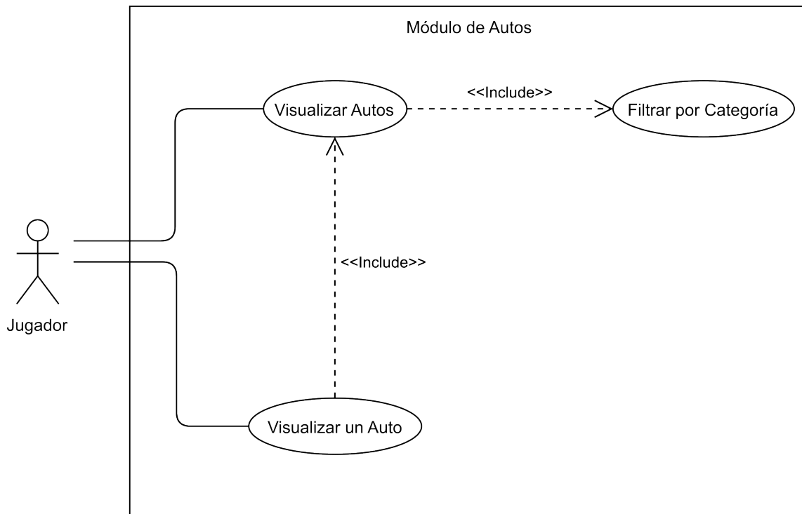
Figura 6.3: Segundo diagrama de casos de uso del módulo de autos
