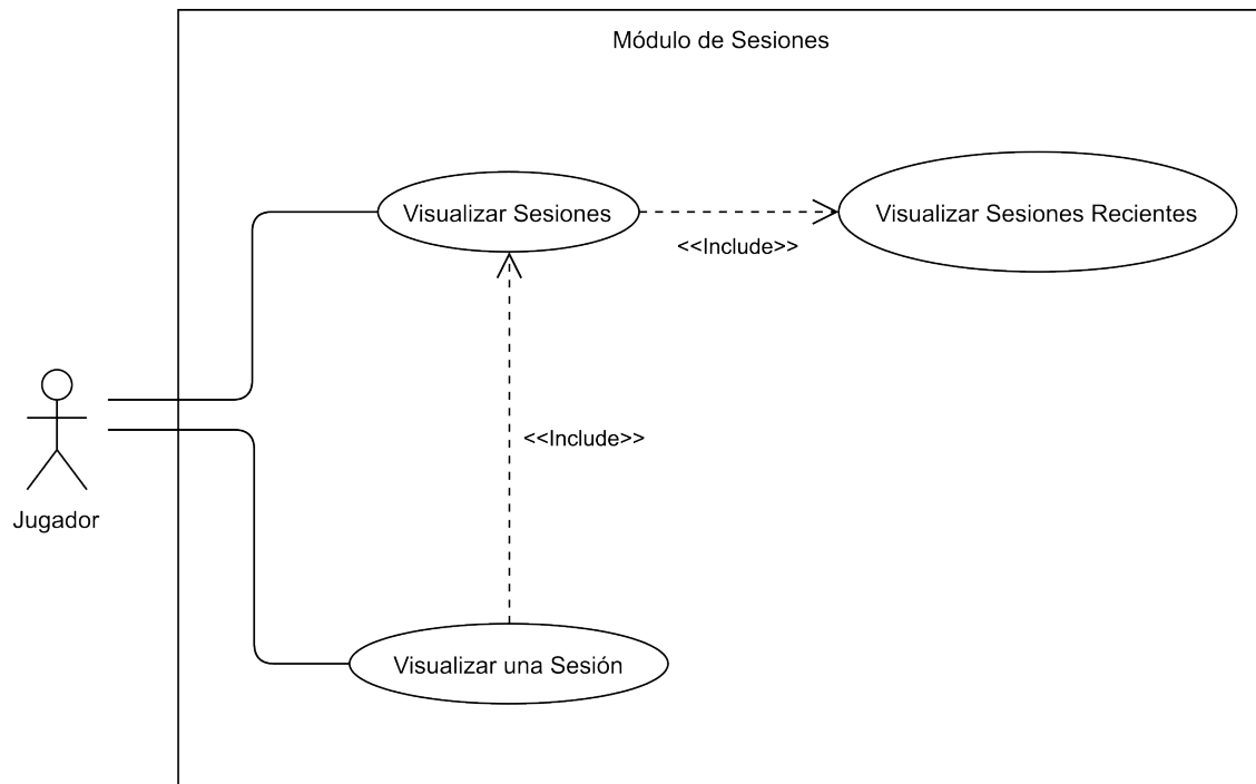
Figura 6.9: Segundo diagrama de casos de uso del módulo de sesiones
